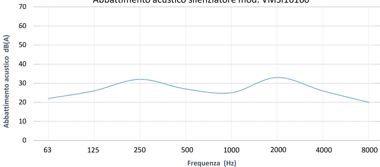
Abbattimento acustico silenziatore mod. VMSI16160
