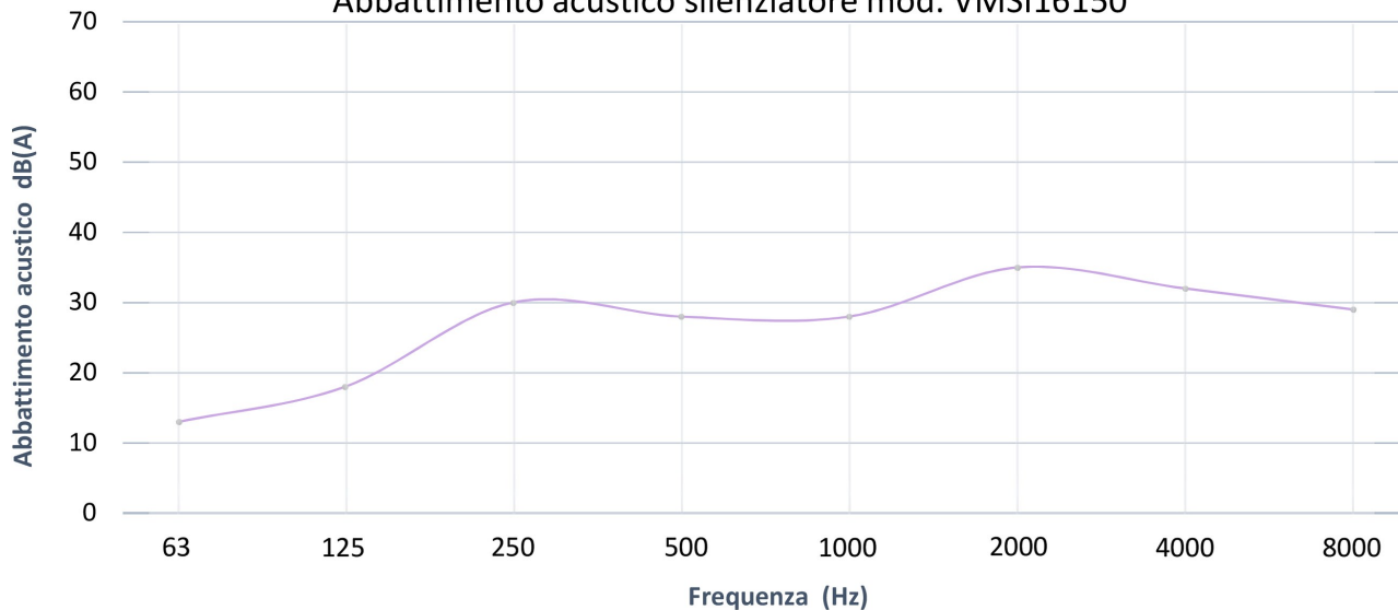
Abbattimento acustico silenziatore mod. VMSI16150
