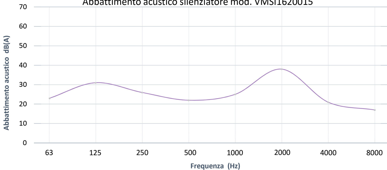
Abbattimento acustico silenziatore mod. VMSI1620015
