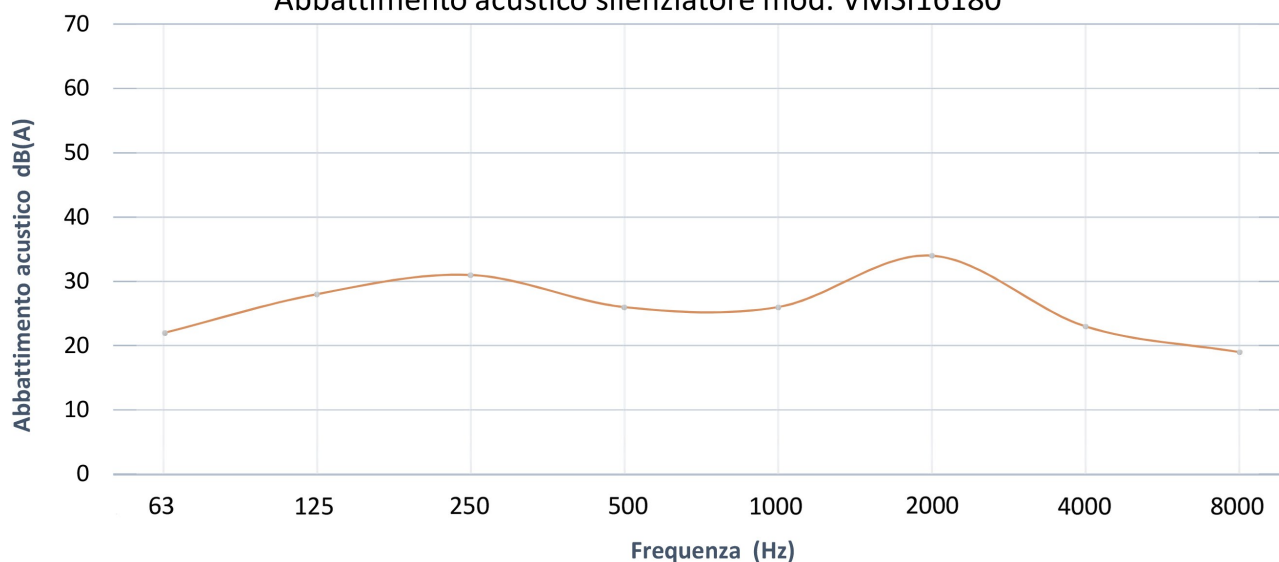
Abbattimento acustico silenziatore mod. VMSI16180
