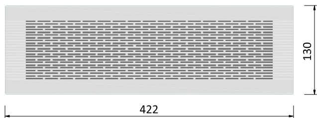
VISTA FRONTALE
